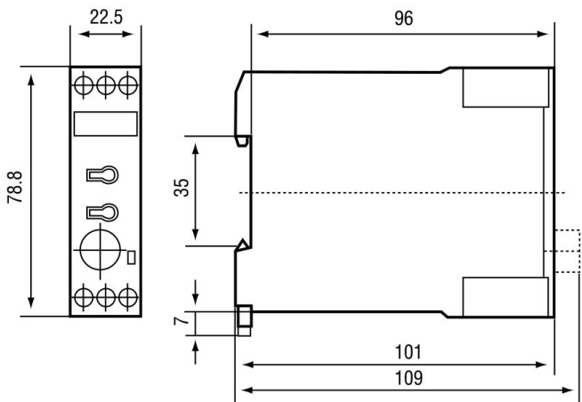
RZ7-FS (1 C/O)
