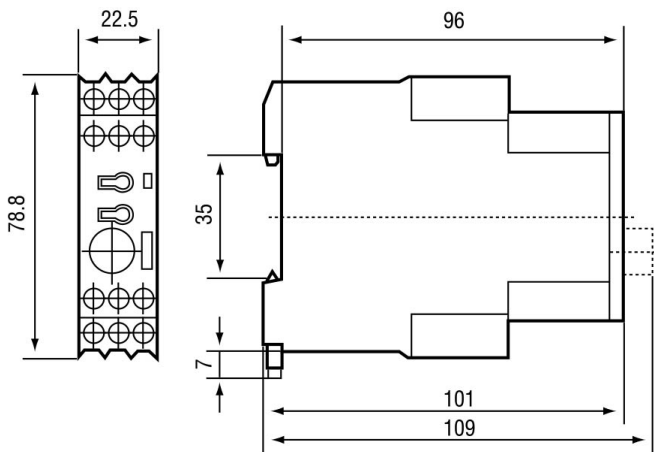
RZ7-FS (2 C/O)
